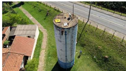
Foto 8 - Escada, tubulação de alimentação e extravasor.
