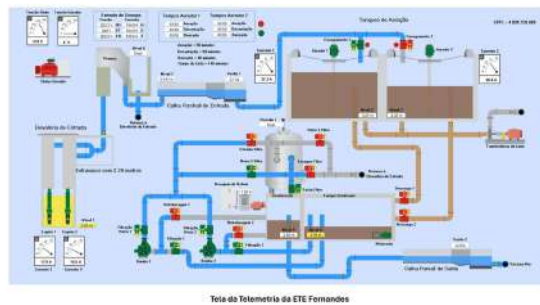
Foto 7 - Tela do sistema de telemetria da ETE Fernandes.
