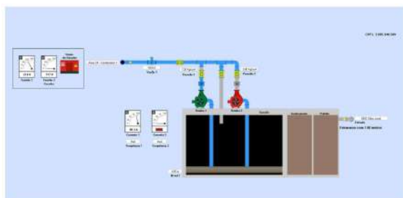
Foto 7 - Tela do sistema de telemetria da EEE Corrupira.
