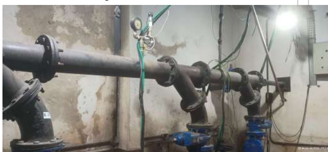
Foto 27 - Barrilete de recalque da antiga casa de bombas.
