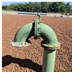
Foto 4 - Tubulação de ventilação
