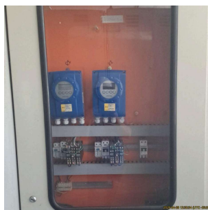
Foto 15 - Display dos medidores de vazão da captação
