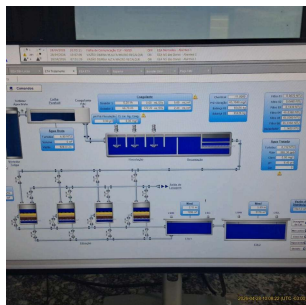
Foto 1 - CCO - Tela mostrando a medição de vazão na entrada da ETA
