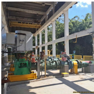
Foto 10 - Vista interna da captação
