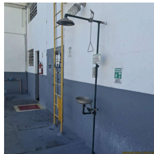
Foto 25 - Chuveiro de emergência
