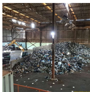
Foto 2 - Entrada de resíduos oriundos da coleta domiciliar e equipamento rasga-sacos
