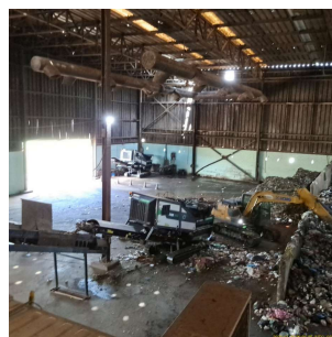
Foto 4 - Rasga-sacos
