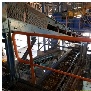
Foto 6 - Esteira de separação de materiais ferrosos
