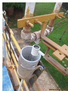
Foto 12 - Dosagem de flúor
