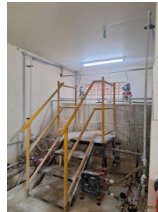
Foto 25 - Tanque de preparo de cal
