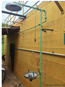
Foto 24 - Chuveiro de emergência - área externa
