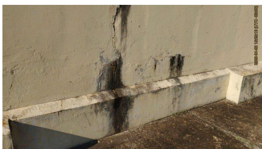
Foto 1 - Ponto com vazamento na parede do reservatório.
