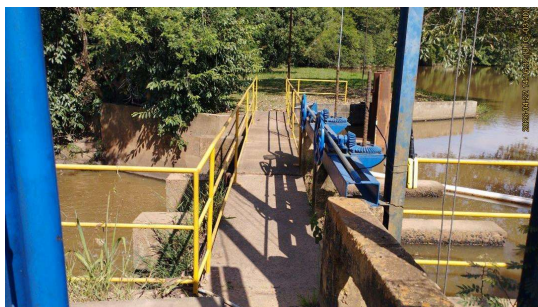
Foto 5 - Vista geral do ponto de captação na Represa Santa Alice.
