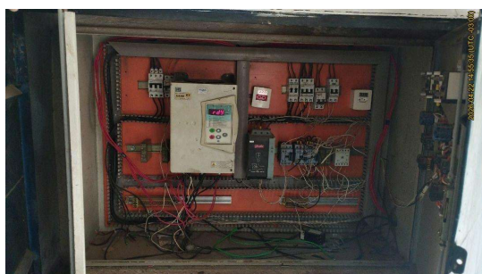
Foto 7 - Detalhe do painel elétrico.
