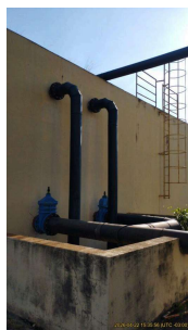
Foto 11 - Detalhe dos tubos extravasores do reservatório.
