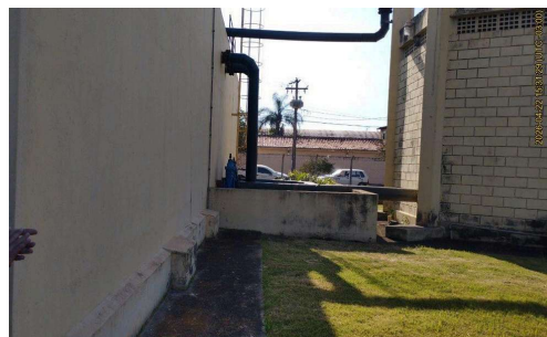
Foto 10 - Tubulação de saída do reservatório, conectada à elevatória de água instalada na edificação sob o reservatório elevado.
