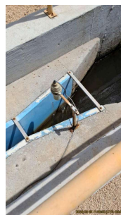
Foto 19 - Calha Parshall e macromedidor de vazão na saída do efluente após o tratamento.
