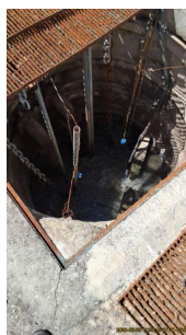
Foto 2 - Poço de sucção sem proteção.
