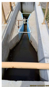
Foto 20 - Estrutura de saída do efluente tratado destinada ao lançamento no corpo receptor.
