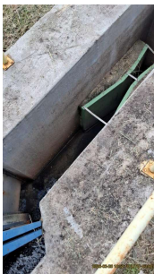
Foto 4 - Calha Parshall para medição de vazão.
