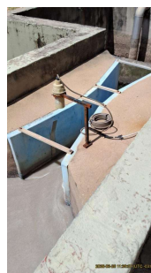
Foto 9 - Calha Parshall e macromedidor de vazão.
