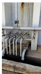
Foto 12 - Ponto de descarga de lodo.
