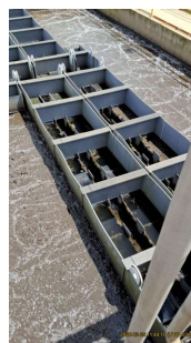
Foto 17 - Detalhe das calhas do decantador, responsáveis pela coleta e direcionamento do efluente clarificado.
