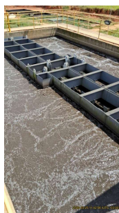
Foto 16 - Vista geral das câmaras de tratamento, onde ocorre a remoção de sólidos e a estabilização do efluente.
