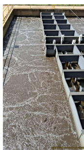
Foto 14 - Câmara de aeriação do sistema de lodos ativados, com destaque para a calha central do decantador secundário destinada à coleta do efluente clarificado.
