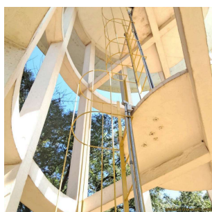
Foto 3 - Escada de acesso e guarda-corpo
