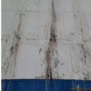
Foto 5 - Vista 5 - Vazamentos na parede do reservatório
