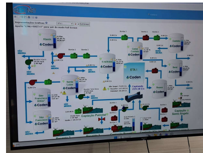
Foto 6 - Medição de nível (telemetria)
