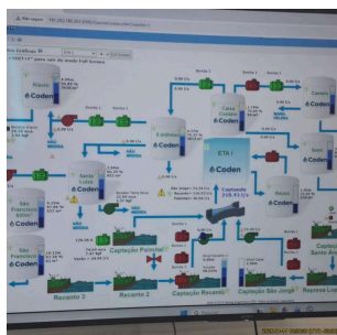
Foto 5 - Medição de nível (telemetria)
