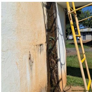
Foto 3 - Vista 3 - Vazamento na junta do decantador 1
