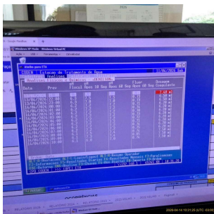
Foto 13 - Planilhas de análises de controle do processo
