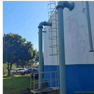
Foto 4 - Tubulação de entrada de água e extravasor
