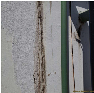
Foto 1 - Vista 1 - Vazamento na parede do decantador 1
