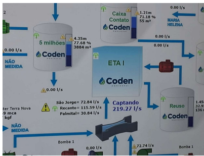
Foto 1 - Telemetria com ausência de leitura da vazão dos reservatórios 5000 e Semienterrado ETA
