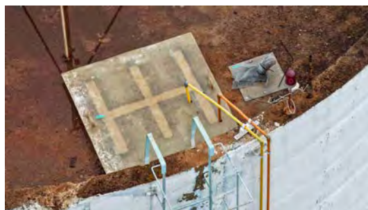
Foto 10 - Tampa de inspeção, local de aplicação de produtos químicos e tubulação de ventilação com tela.
