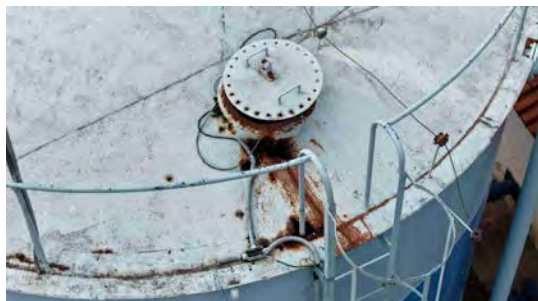
Foto 7 - Aberturas ocasionadas por corrosão.
