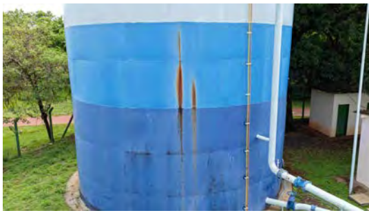
Foto 1 - Início de corrosão na lateral do reservatório.
