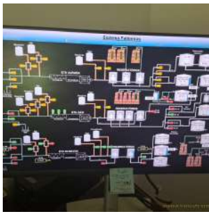
Foto 26 - Tela CCO (em desenvolvimento)
