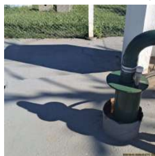
Foto 4 - Tubo de medição de nível e laje de proteção
