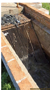
Foto 3 - Segunda unidade de gradeamento grosseiro do sistema.
