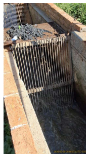
Foto 2 - Primeira unidade de gradeamento grosseiro do sistema.
