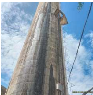
Foto 7 - Vista geral do reservatório elevado.
