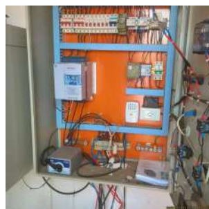
Foto 17 - Pannel elétrico e de comando da elevatória (com soft starter)
