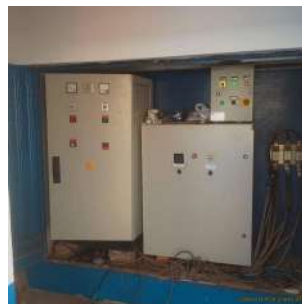
Foto 14 - Painéis elétricos e de comando dos equipamentos e do poço.
