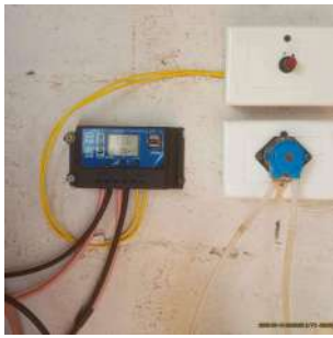
Foto 21 - Bomba dosadora de hipoclorito.
