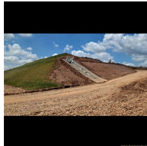
Foto 4 - Sistema de drenagem
