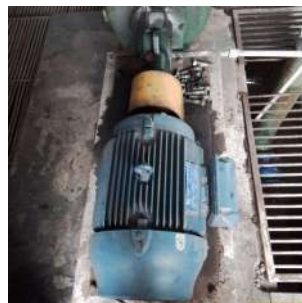
Foto 4 - Conjunto motobomba 1
