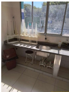
Foto 17 - Laboratório de análises físico-químicas, onde são realizados testes de sólidos sedimentáveis (cone Imhoff), pH e condutividade. Ensaio mais complexos são feitos em laboratório parceiro ou em outra ETE do município.
