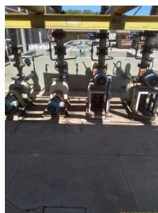
Foto 10 - Motobombas utilizadas no recalque do esgoto bruto para tratamento.
