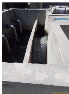
Foto 7 - Sistema de recalque do esgoto bruto para as câmaras de tratamento.
