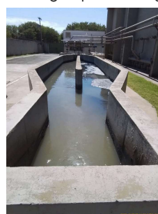
Foto 5 - Passagem do esgoto bruto.
