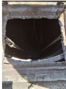
Foto 4 - Bomba submersa e peneira para retenção de sólidos grosseiros.
