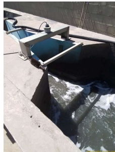
Foto 30 - Calha Parshall e medidor de vazão.
