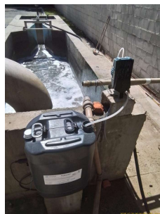
Foto 29 - Ponto de adição de antiespumante.
