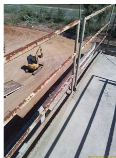
Foto 4 - Guarda-corpo com diversos pontos de oxidação, incluindo áreas com corrosão.
