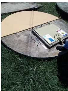
Foto 5 - Tampa de proteção do acesso à bomba submersa e à peneira.
