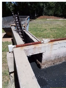
Foto 5 - Grade mecanizada do tipo rosca sem-fim para retirada de sólidos.
