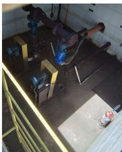
Foto 8 - Interior da estação elevatória, onde se encontram as motobombas de recalque.
