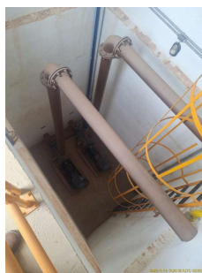
Foto 3 - Escada com guarda-corpos para acesso aos conjuntos motobomba e dois conjuntos instalados
