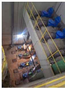
Foto 5 - Quatro conjuntos motobomba instalados
