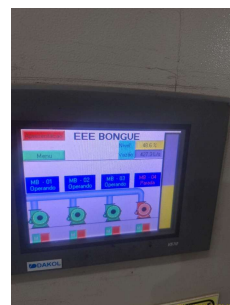
Foto 4 - Visor do painel da bombas, três em operação e uma em espera
