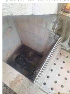
Foto 7 - Gradeamento entrada do poço úmido
