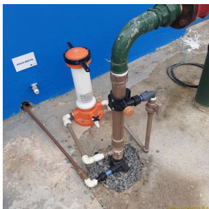
Foto 4 - Ponto de aplicação de cloro e flúor na água bruta. Para aplicação de cloro é utilizado um sistema de pastilhas.
