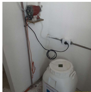
Foto 8 - Tanque de armazenamento e bomba dosadora de flúor.
