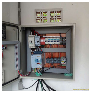
Foto 10 - Vista interna do painel elétrico.
