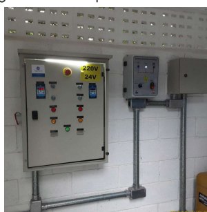
Foto 4 - Painéis elétricos.
