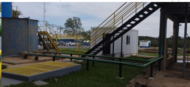
Foto 12 - ETA-5.2 - ETA JUNDIAQUARA: Novo sistema de tratamento de lodo - Tubulação do sistema e pontos de aplicação de polímero.
