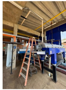
Foto 26 - Centrífugas
