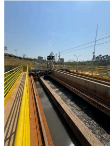
Foto 8 - Desarenador
