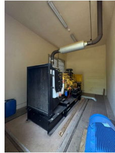
Foto 28 - Moto-gerador
