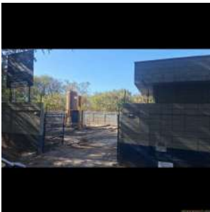
Foto 2 - Visão geral - portão e entrada da Estação Elevatória de Esgoto
