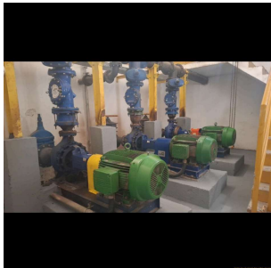
Foto 7 - Conjuntos motobombas
