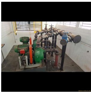
Foto 9 - Conjuntos motobombas
