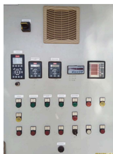
Foto 11 - Painel das centrífugas
