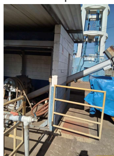
Foto 8 - Transportador helicoidal para lodo
