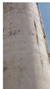
Foto 10 - Vazamento na estrutura do Reservatório Elevado Vila Brasil em Santa Bárbara DOeste
