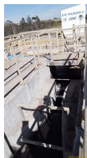
Foto 10 - Calha Parshall da ETE Toledos II em Santa Bárbara DOeste
