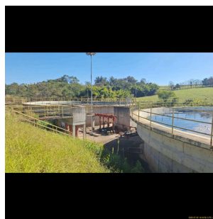
Foto 18 - Recalque do lodo ao centro
