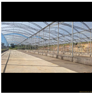
Foto 26 - Estufa para secagem do lodo - ainda não sendo utilizada
