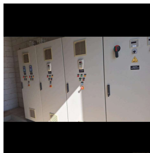
Foto 14 - Painéis elétricos dos sopradores
