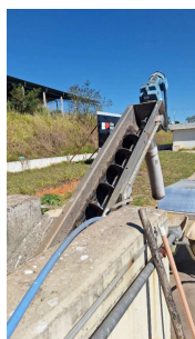
Foto 3 - Rosca helicoidal - remoção de areia do tratamento preliminar
