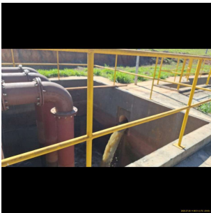
Foto 1 - Esgoto Bruto, pós desarenador em poço pulmão para recalque à ETE Rio Sorocaba
