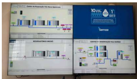
Foto 14 - Tela do Centro de Controle Operacional. O nível dos reservatórios é monitorado por telemetria.
