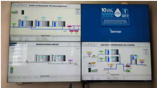
Foto 7 - Tela do Centro de Controle Operacional. O nível dos reservatórios é monitorado por telemetria.
