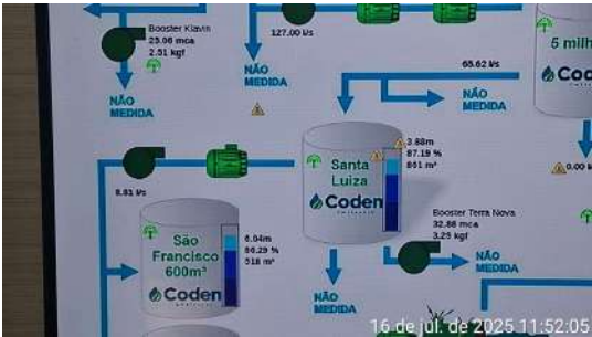
Foto 6 - Telemetria
