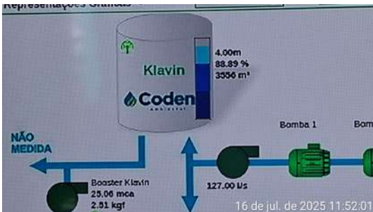
Foto 5 - Telemetria
