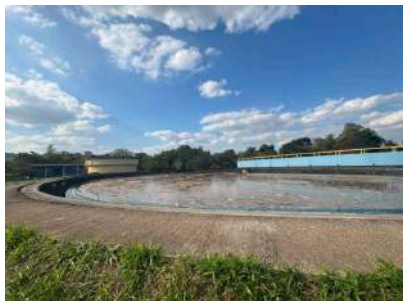
Foto 17 - Decantador secundário
