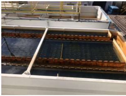
Foto 1 - Vertedores
