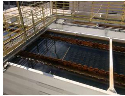
Foto 2 - Vertedores
