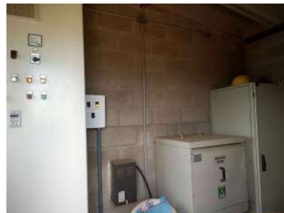
Foto 7 - Painel de comando e controle
