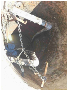
Foto 7 - Poço de sucção - um conjunto moto bomba instalado
