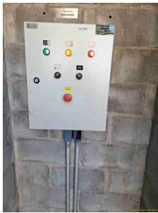
Foto 3 - Paineleletrico dentro de abrigo
