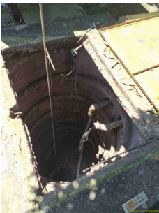
Foto 2 - Dois conjuntos motobomba instalados - um içado em cabo de aço e outro por corrente
