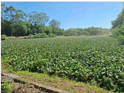
Foto 4 - ETE São Jorge - lagoa facultativa - visão geral - aguapés na lagoa
