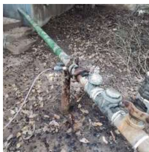
Foto 2 - Vazamento na tubulação da Captação subterrânea Poço 1 em Ipeúna
