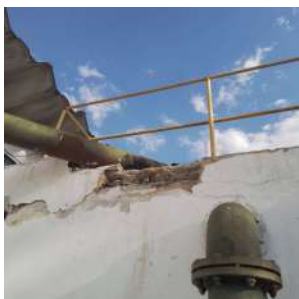
Foto 5 - Danos estruturais na junção entre a parede e a laje
