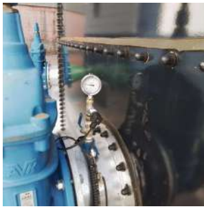
Foto 7 - Manômetro
