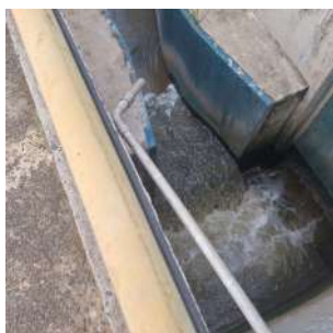
Foto 21 - Dosagem de antiespumante na saída do efluente tratado
