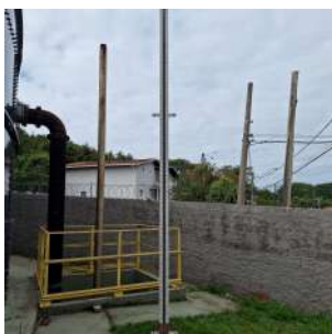
Foto 1 - Medidor de nível mecânico -
