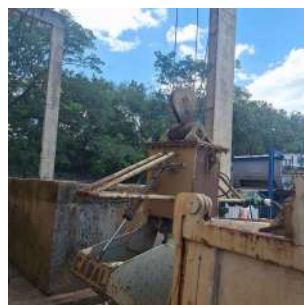
Foto 6 - Sistema para remoção de areia sem paralisar ete
