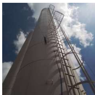
Foto 2 - Descida do cabeamento do SPDA na lateral da escada..
