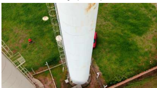
Foto 8 - Vista aérea da base do reservatório antigo (branco).
