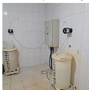
Foto 6 - Casa de química - dosagem de produtos - Poço Baggio
