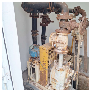
Foto 4 - Conjunto motobomba instalado - EEEB Pazoto
