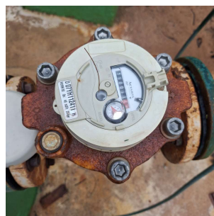
Foto 3 - Macromedidor - Poço Baggio
