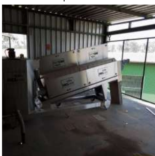
Foto 3 - Skid para adensamento e tratamento do lodo.
