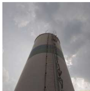
Foto 2 - Cabo de descida do para-raios
