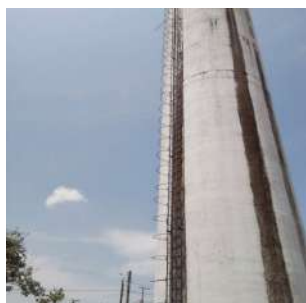
Foto 1 - Falta de proteção vertical na escada marinho Reservatório elevado do Jardim Módolo em Cordeirópolis
