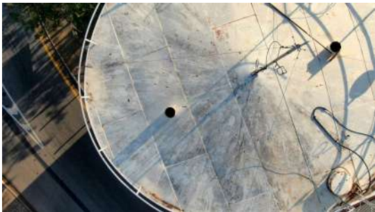
Foto 1 - Reservatório Country Club - ausência de telas de proteção
