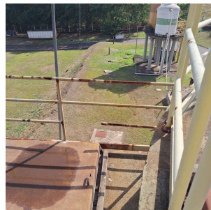
Foto 2 - Guarda-corpos quebrado
