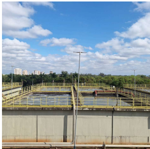
Foto 6 - Um módulo com quatro células _ lodos ativados _
