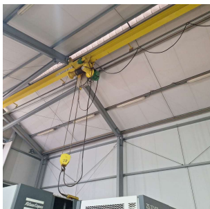
Foto 10 - Guindaste de para retiradas para manutenção dos sopradores
