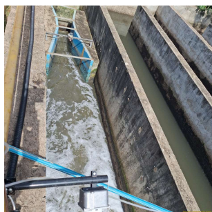
Foto 1 - Macromedidor na saída
