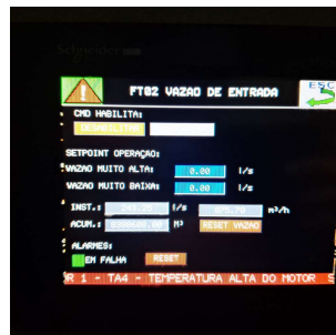
Foto 11 - Monitoramento da vazão de entrada do esgoto
