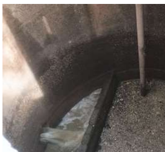
Foto 9 - Vista interna do poço de sucção.
