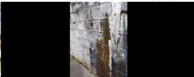
Foto 2 - Vazamentos na estrutura do Reservatório Semienterrado Maranguape em Atibaia
