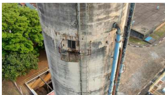
Foto 2 - Guarda-corpos inadequados do Reservatório Elevado da ETA Cerejeiras em Atibaia
