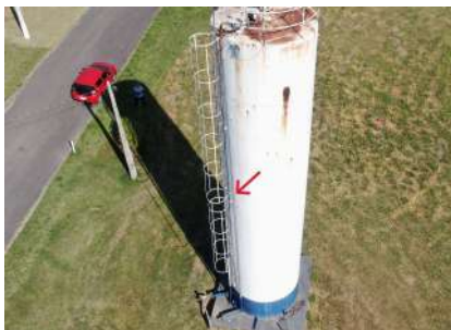
Foto 1 - Detalhe do tubo extravasor indicado pela seta vermelha.
