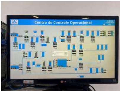
Foto 1 - CCO do DAAE, exibindo o sistema de telemetria.
