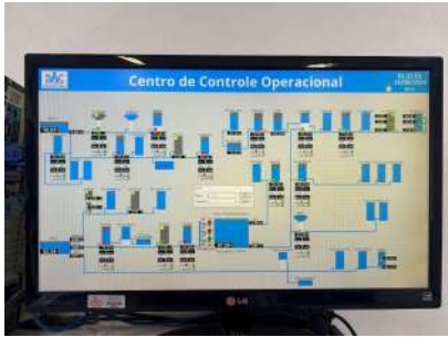
Foto 1 - CCO do DAAE exibindo sistema de telemetria.
