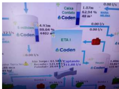
Foto 1 - Detalhe da telemetria com vazão ETA
