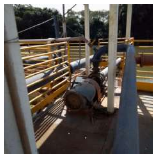
Foto 4 - Captação João de Souza em São José do Rio Pardo
