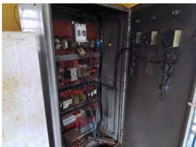
Foto 5 - Detalhe interno do painel elétrico da EEAT Vila Bandeirantes.
