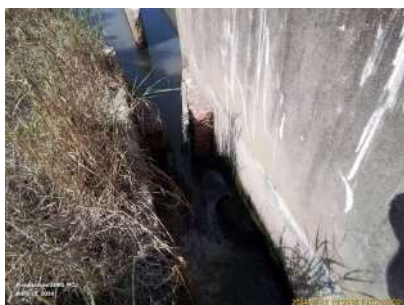
Foto 1 - Calha Parshall do preliminar quebrada.
