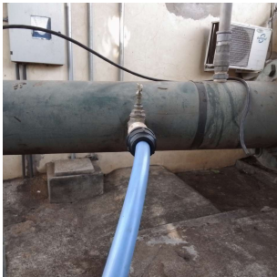
Foto 4 - Tomada para coleta de água bruta do poço Pernambuco
