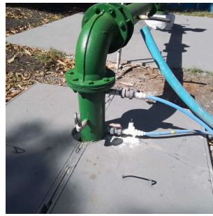
Foto 8 - Ponto de dosagem de cloro e flúor
