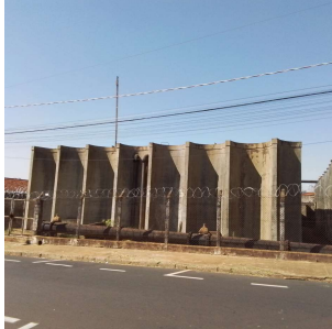
Foto 1 - Reservatório Maranhão I
