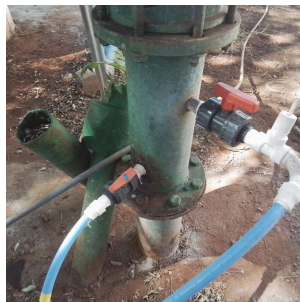
Foto 4 - Ponto de dosagem de cloro e flúor
