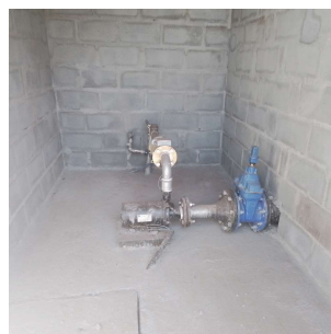
Foto 2 - Conjunto motor-bomba
