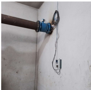
Foto 10 - Medidor de vazão
