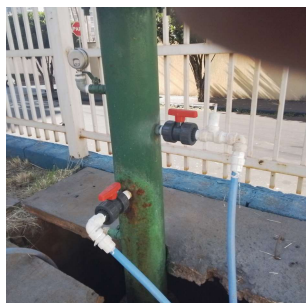
Foto 7 - Ponto de dosagem de cloro e flúor
