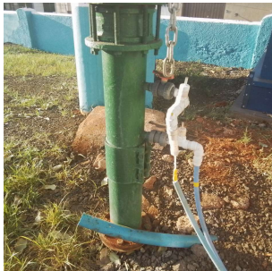
Foto 5 - Ponto de aplicação da dosagem de cloro e flúor
