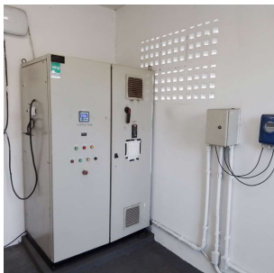
Foto 11 - Painel de comando e controle
