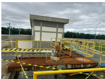
Foto 1 - Guarda-corpos com oxidação avançada
