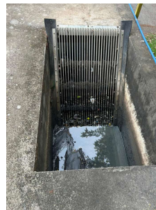
Foto 10 - Gradeamento
