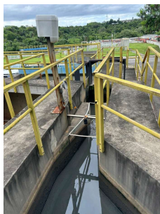
Foto 11 - Canal de entrada
