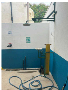
Foto 7 - Chuveiro de emergência
