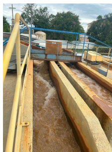
Foto 20 - Entrada de água bruta
