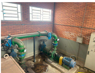
Foto 1 - Conjuntos moto-bomba
