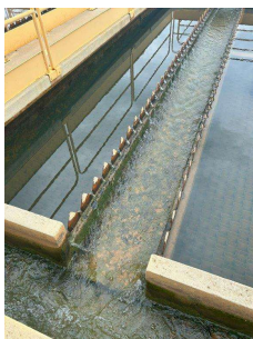
Foto 19 - Decantador
