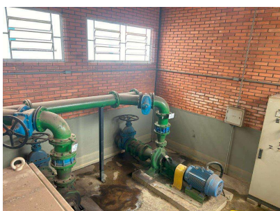
Foto 1 - Drenagem inadequada das gaxetas
